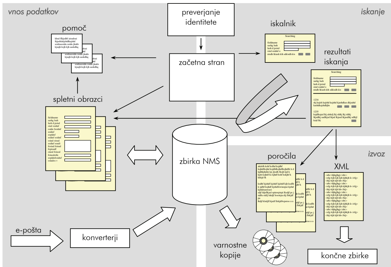
Slika 2 Shematski prikaz funkcij sistema. Enostavne puščice predstavljajo možna dejanja uporabnikov, široke puščice na tok podatkov.
