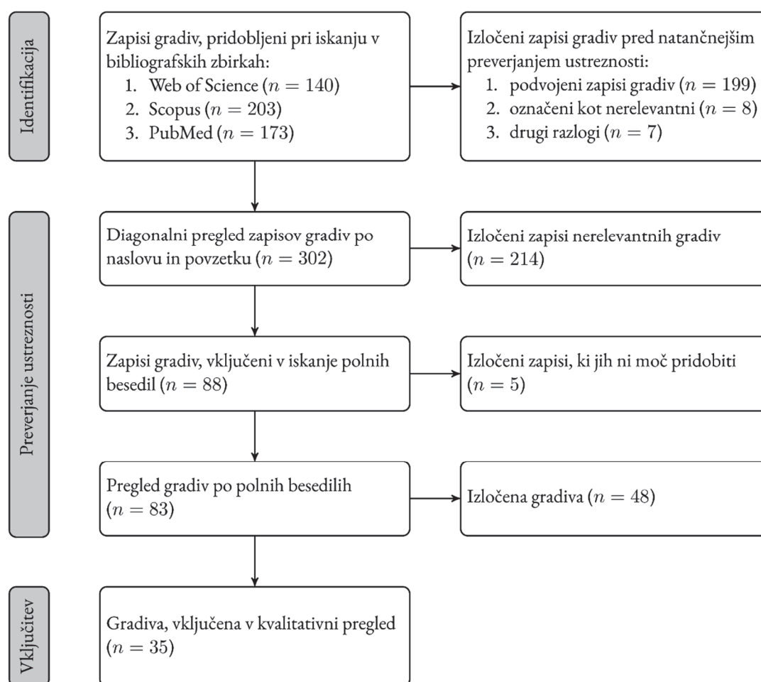
Slika 3 PRISMA diagram poteka iskanja in izbora gradiva.
